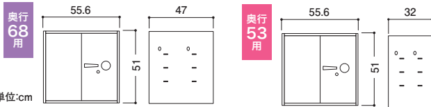
ダイヤル錠
