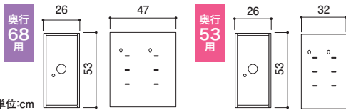
テンキー錠
